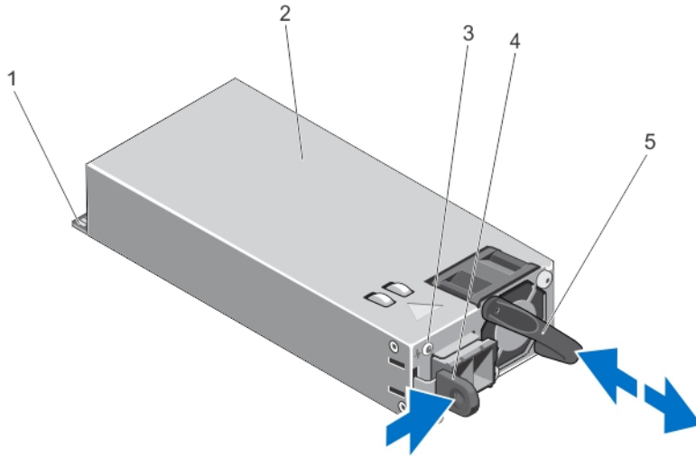
图 43: 卸下和安装直流电源设备
