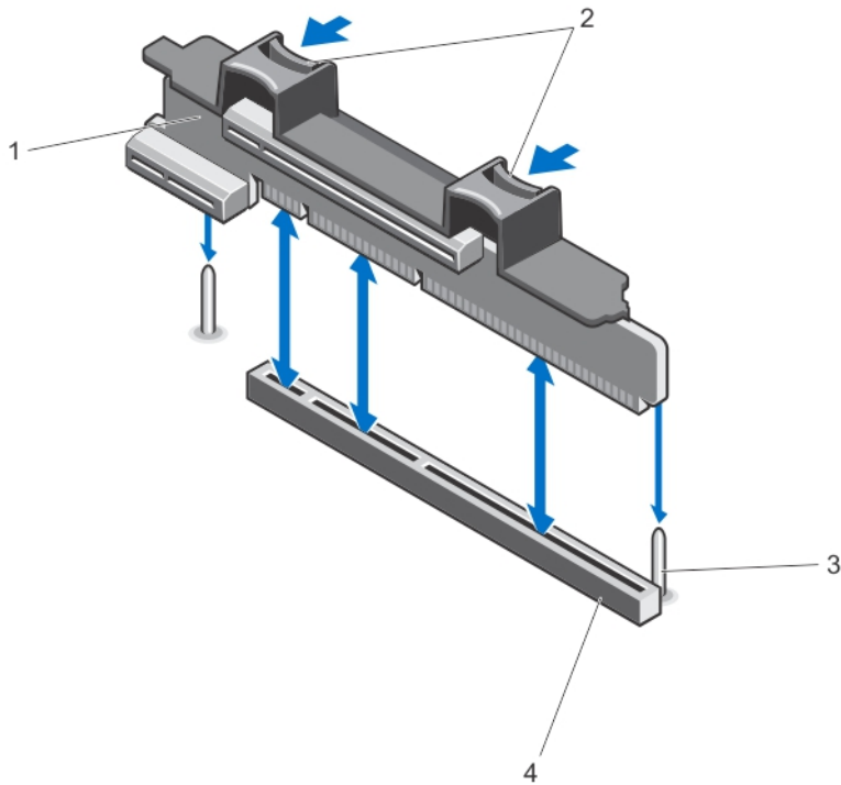
图 32: 卸下和安装扩充卡提升板 1
