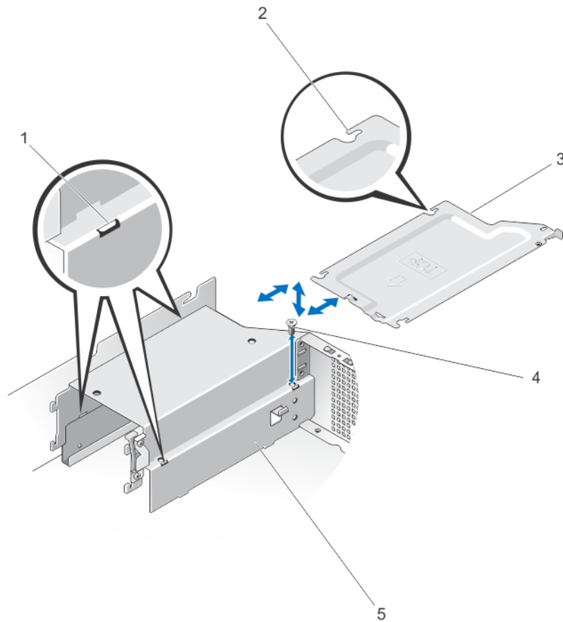
图 49: 卸下并安装冗余电源设备装置分隔架
