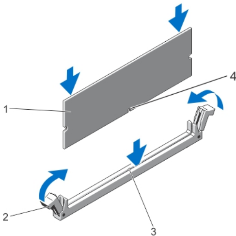
图 19: 安装内存模块
