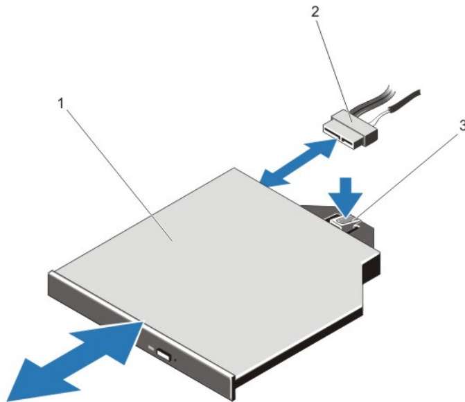
图 27: 卸下和安装光盘驱动器
