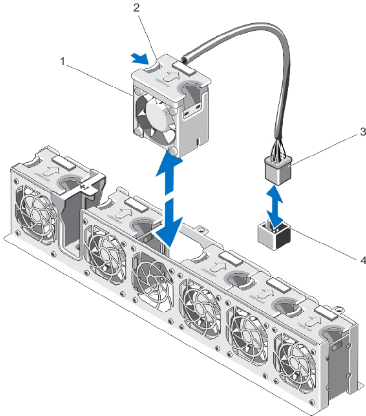
图 28: 卸下和安装冷却风扇
