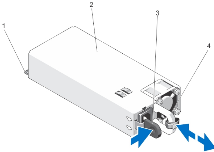
图 40: 卸下和安装交流电源设备
