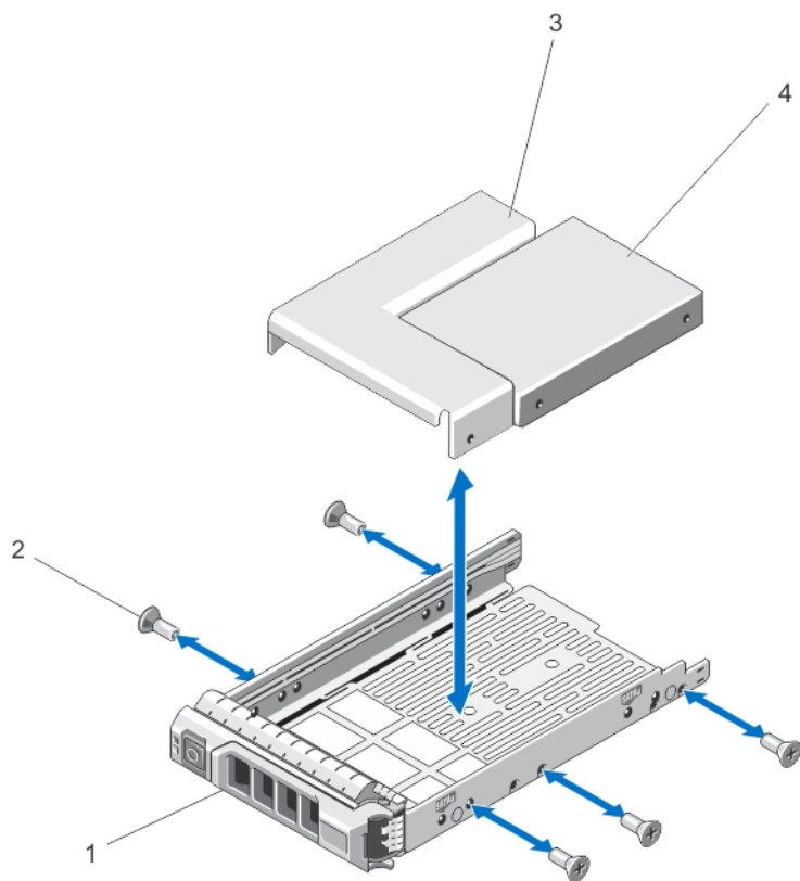
图 26: 卸下并安装硬盘驱动器适配器到 3.5 英寸硬盘驱动器托盘中
