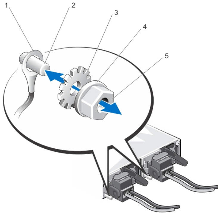
图 41: 安装和连接安全接地线
