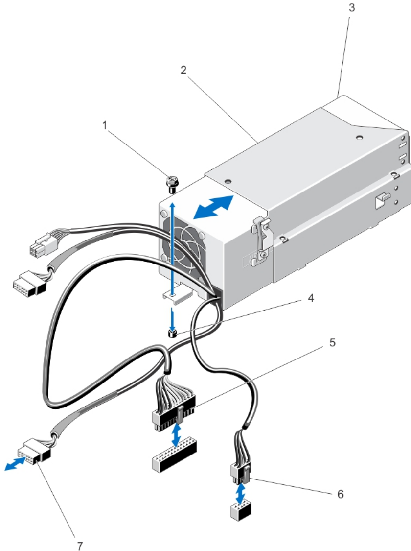
图 48: 卸下和安装非冗余电源设备
