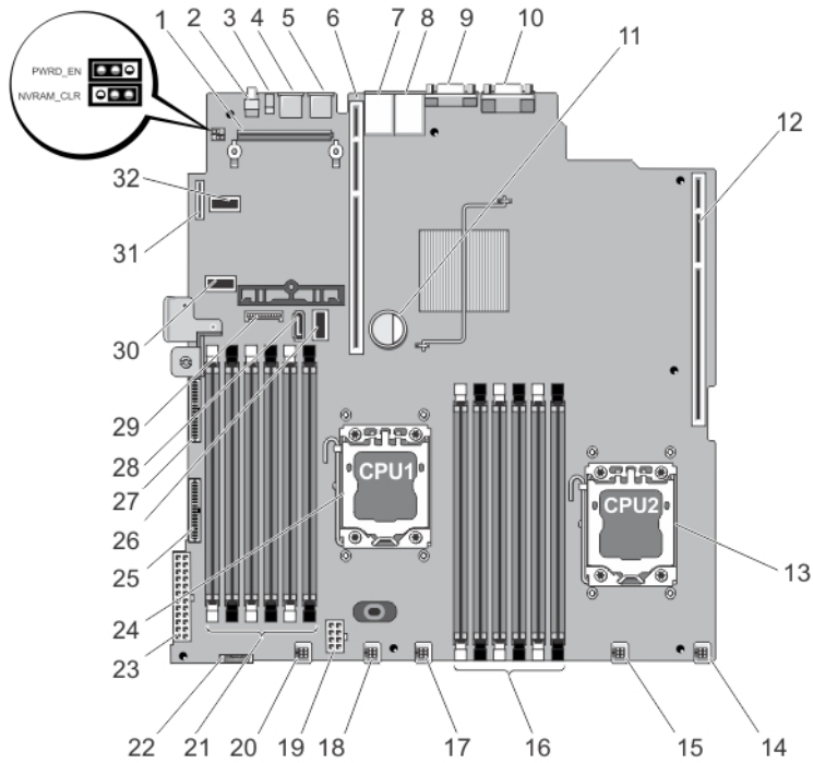
图 56: 系统板连接器和跳线
