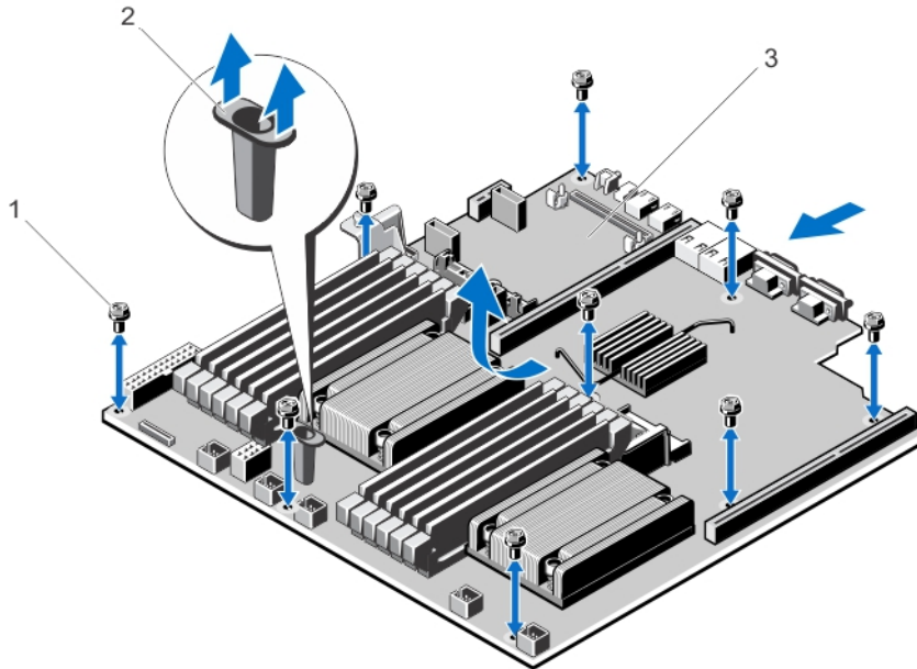
图 55: 卸下和安装系统板
