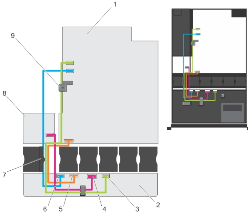
图 52: 冗余 PSU 系统的硬盘驱动器背板的布线图
