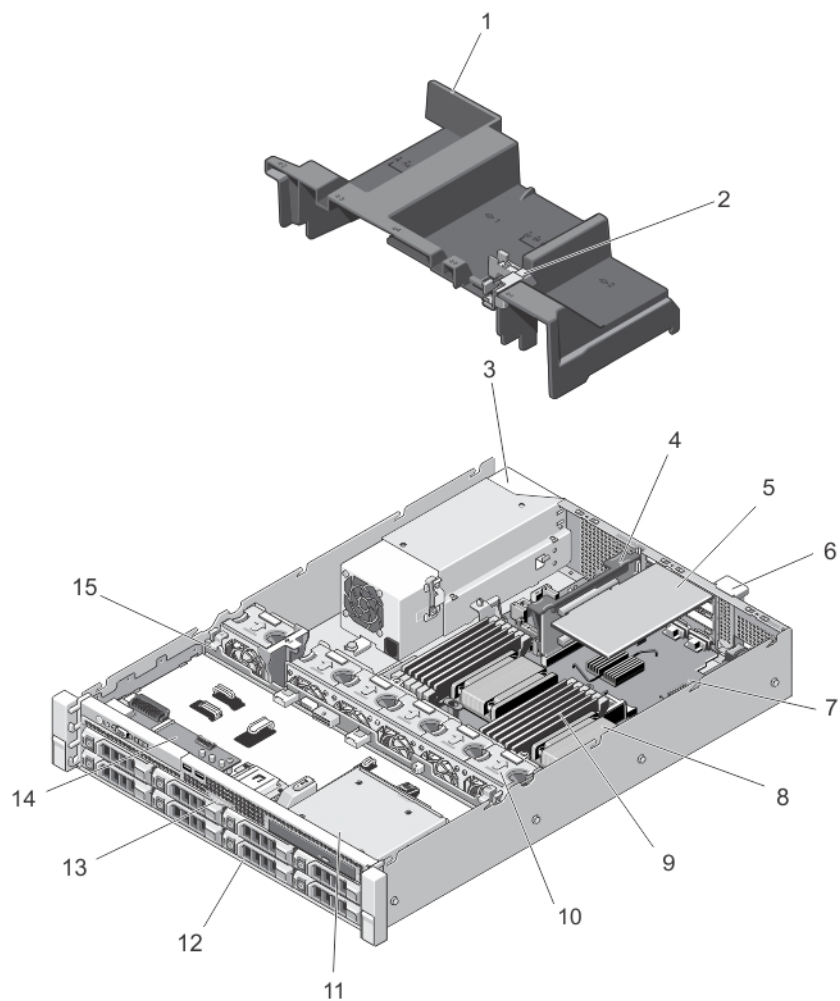
图 14: 系统内部组件—非冗余电源设备机箱
