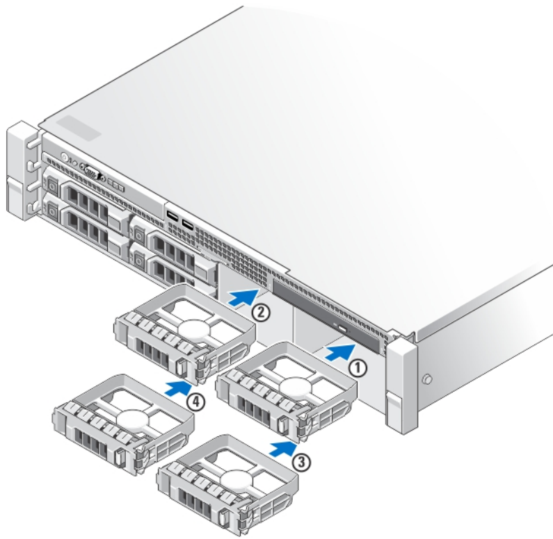
图 21: 硬盘驱动器挡片安装顺序
