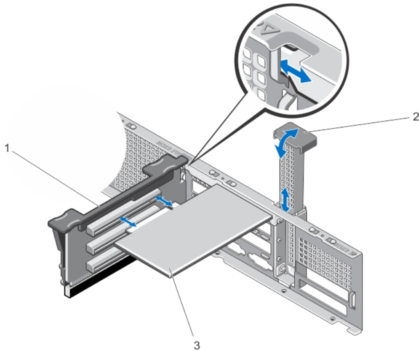
图 31: 从扩充卡提升板 2 处卸下并安装扩充卡
