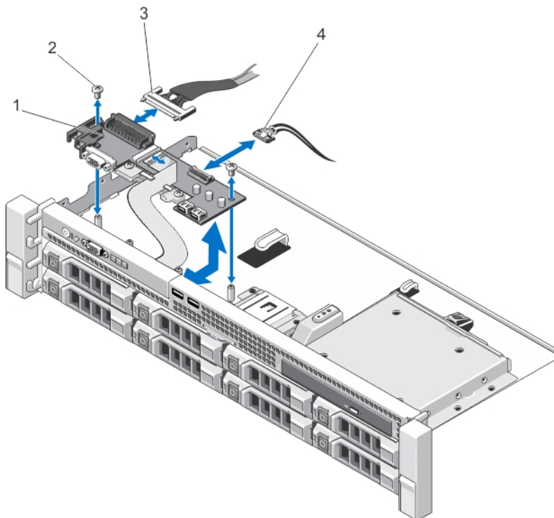
图 54: 卸下和安装控制面板
