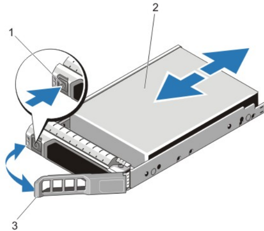
图 23: 卸下和安装热置换硬盘驱动器
