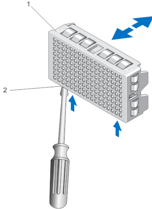
图 22: 卸下和安装双插槽硬盘驱动器挡片
