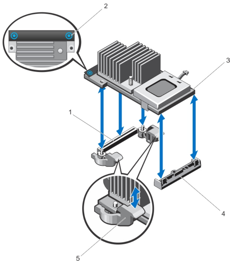
图 37: 卸下和安装集成存储控制器
