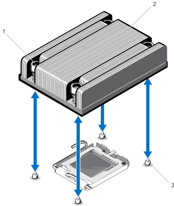
图 38: 卸下和安装散热器
