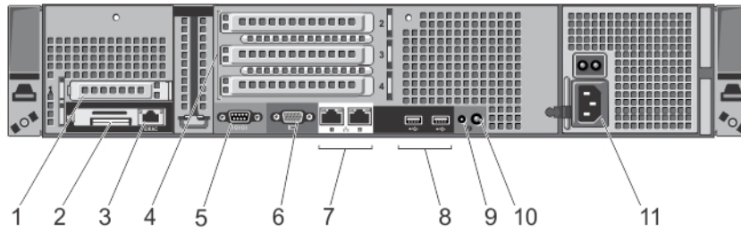
图 6: 背面板部件和指示灯—非冗余电源设备装置机箱
