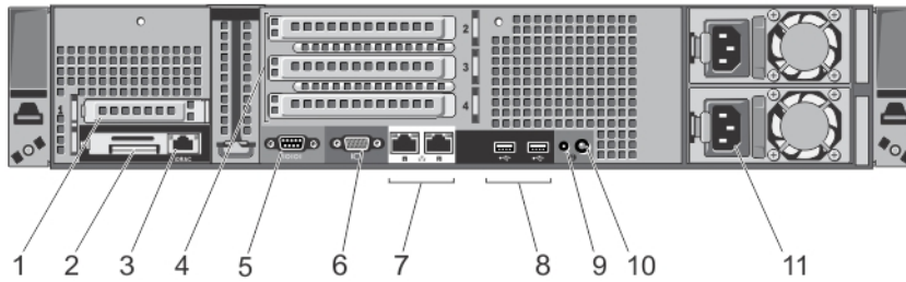
图 5: 背面板部件和指示灯—冗余电源设备装置机箱
