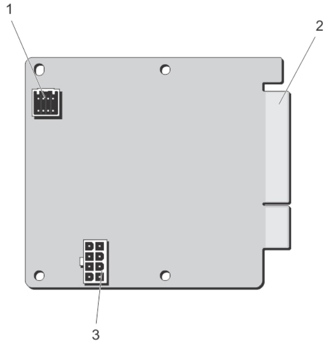
图 46: 配电板连接器
