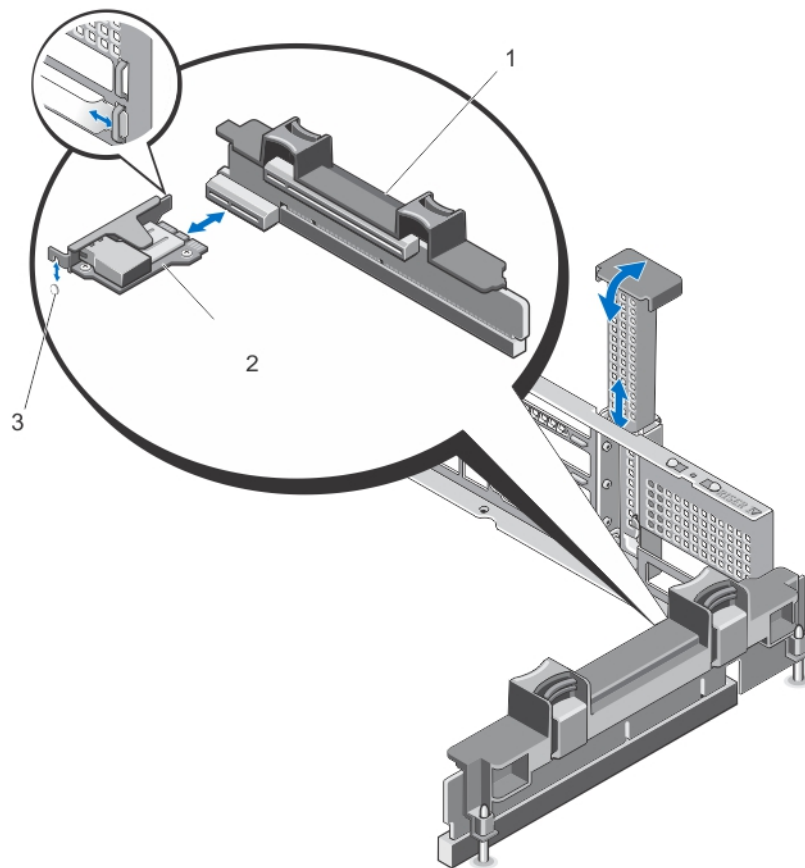
图 34: 卸下和安装 iDRAC 端口卡
