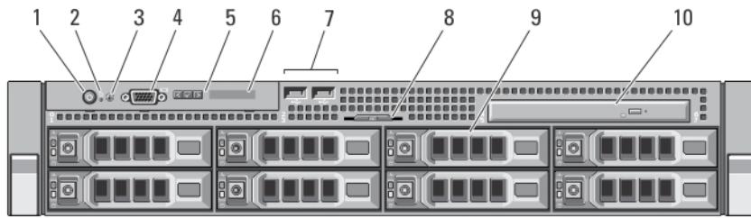
图 1: 前面板部件和指示灯
