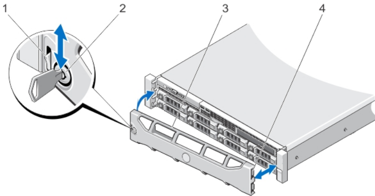
图 11: 安装和卸下前挡板
