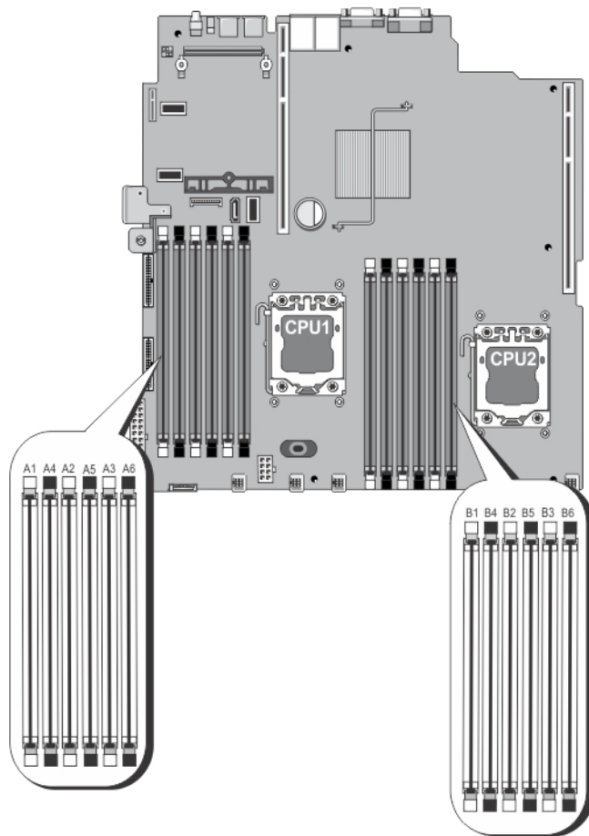
图 16: 内存插槽位置
