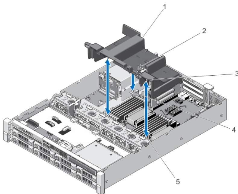
图 15: 卸下和安装冷却导流罩
