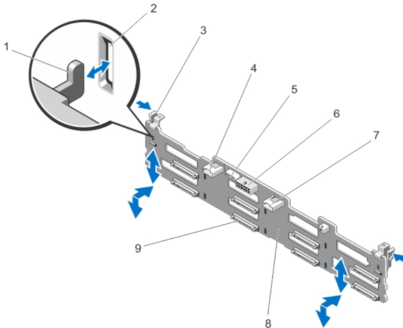
图 51: 卸下和安装硬盘驱动器背板
