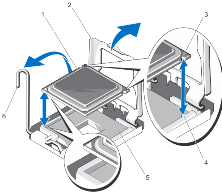
图 39: 卸下和安装处理器
