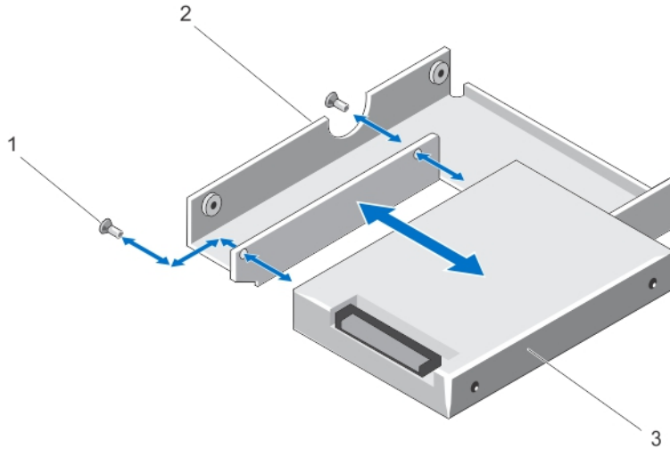
图 24: 从 3.5 英寸硬盘驱动器适配器中卸下和安装 2.5 英寸硬盘驱动器
