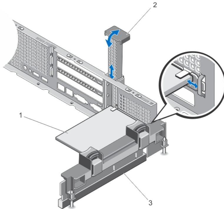
图 30: 从扩充卡提升板 1 处卸下并安装扩充卡
