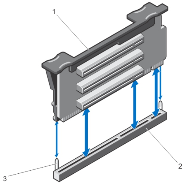
图 33: 卸下和安装扩充卡提升板 2
