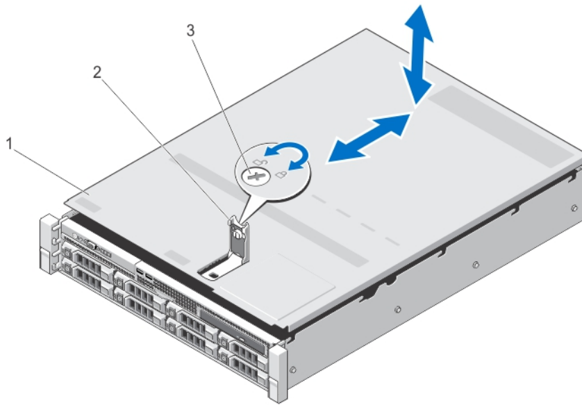
图 12: 打开与合上系统护盖
