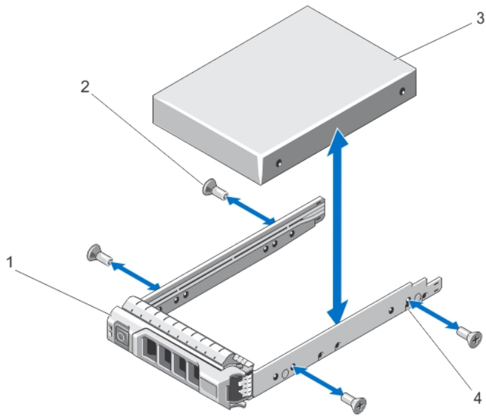
图 25: 在硬盘驱动器托盘中卸下和安装热插拔硬盘驱动器
