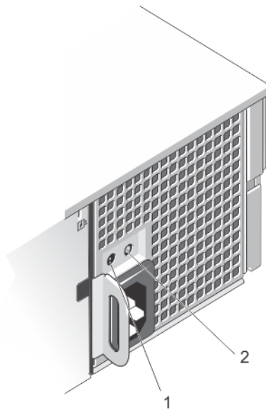
图 10: 非冗余交流电源设备状态指示灯和自我诊断按钮
