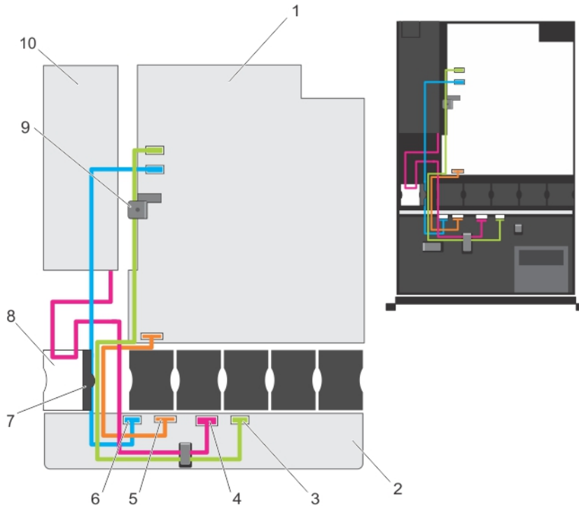
图 53: 非冗余 PSU 系统的硬盘驱动器背板的布线图
