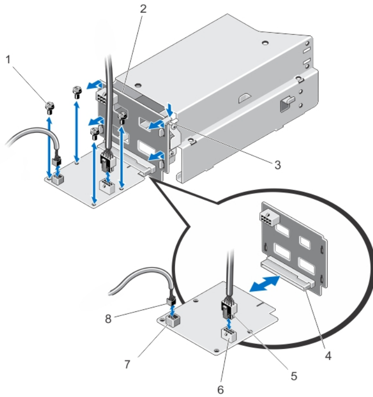
图 45: 卸下和安装配电板
